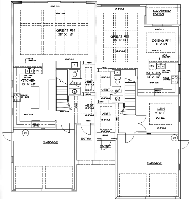
First Floor- 1033 SQ FT 500 NE Wavecrest Way
